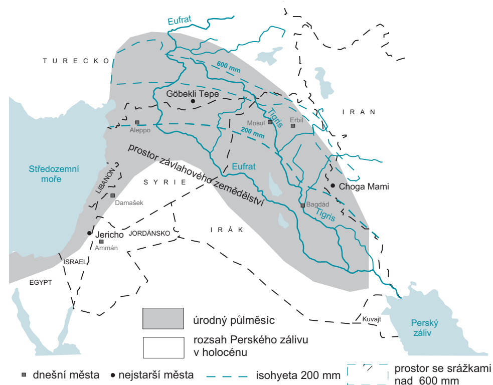
Povodí řek Eufratu a Tigridu, území „úrodného půlměsíce“ a tehdejší srážková činnost
